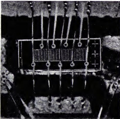
Рис. 2. Структура мощного СВЧ кремниевого транзистора, позволяющего получить мощность 5 вт на частоте 2 Гц (фотография; увеличено в 60 раз). Транзистор содержит 234 эмиттера с размерами 1,5×30 мкм и 18 стабилизирующих резисторов; 18 алюминиевых проволочек соединяют кристалл прибора с выводами.
